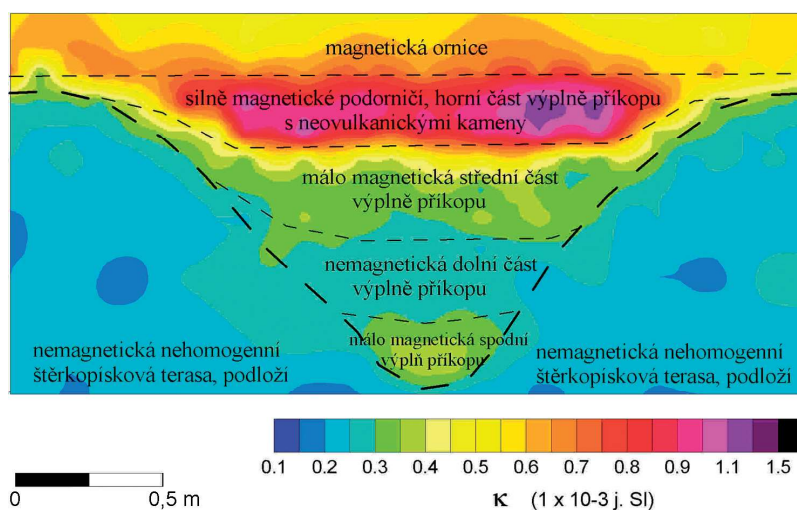
Obr. 12. Ledčice. Výsledek měření magnetické susceptibility na profilu příkopu s rozlišením odlišných výplní – vrstev (zkoumaná plocha: ca 3 x 1,5 m).
